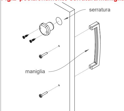
Fig.2 - posizionamento serratura/maniglia
